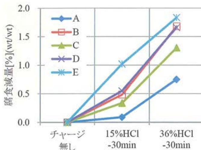
図5：酸浸漬前後の腐食減量
