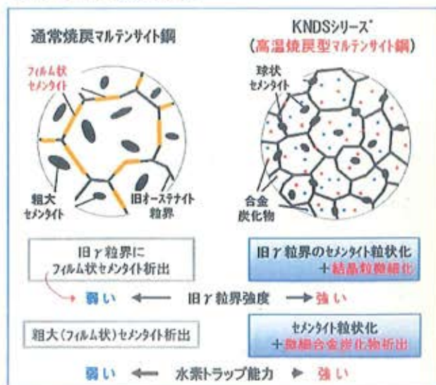
ミクロ組織の比較(イメージ図)
