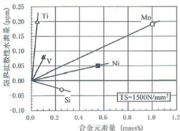
限界水素量に及ぼす化学成分の影響
