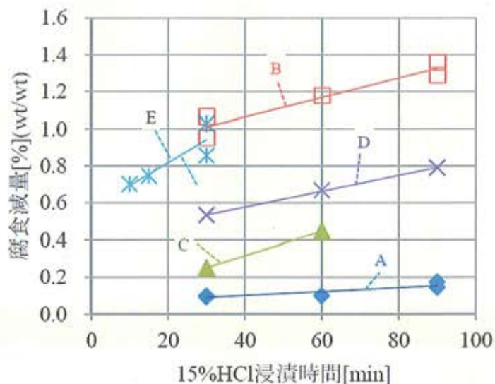
図3. 15% HCl-30min浸漬前後の腐食減量
