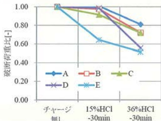
図7. 破断荷重比
