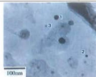
KNDS4の微細析出物(TEM写真) ＜Mo-Ti-V系複合炭化物＞ (1:25nm, 2:15nm, 3:10nm)
