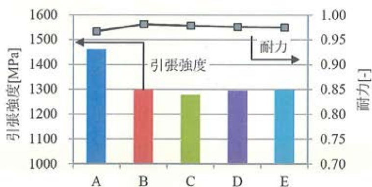
図1. 機械的特性
