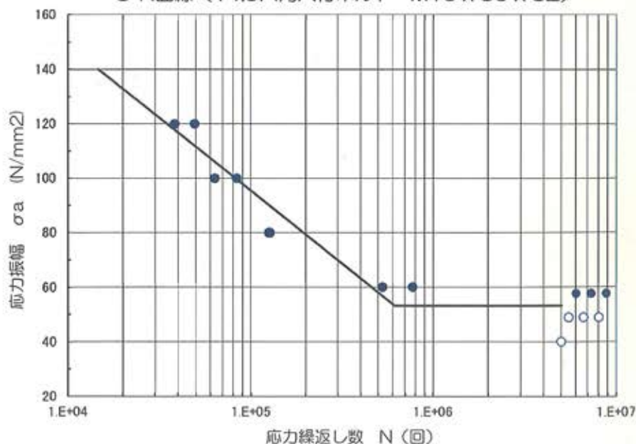
S-N曲線（14.9六角穴付ボルト M10 × 50 × 32）
