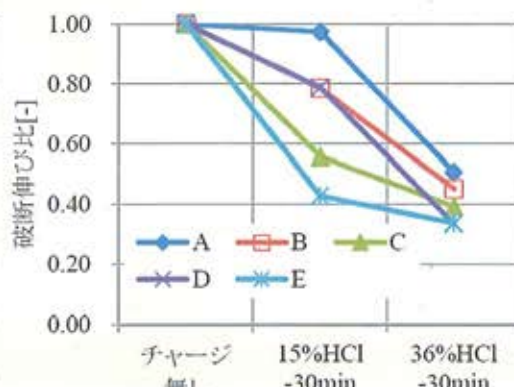
図8. 破断伸び比
