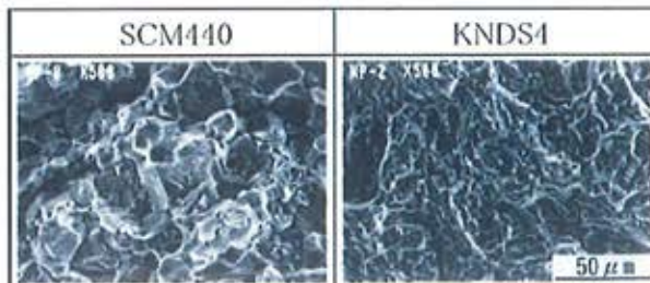
遅れ破壊試験後のSEM破面 (TS=1400N/mm 2 )
