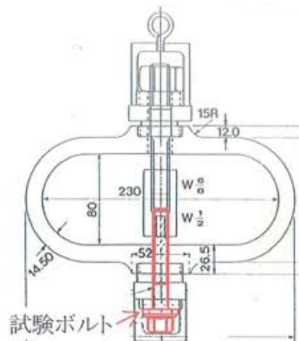
図2. ループ型遅れ破壊試験器
